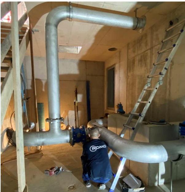
Edelstahl - Rohrleitungsbau im Reservoirkeller
